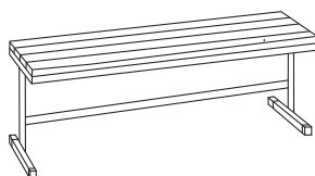
Скамья гардеробная 1000x400x400
