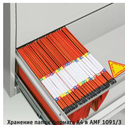
Система полного выдвижения ящиков
