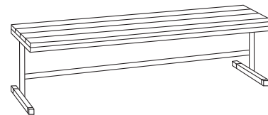
Скамья гардеробная 1500x400x400
