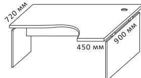
Л.СА-1 Л/Пр 1580x900x755 Л.СА-2 Л/Пр 1380x900x755
