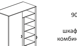
С-ШРК-40 900x400x2050
