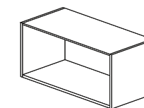
В.А-1 388x359x368 В.А-2 770x359x368
