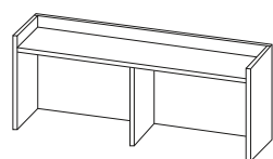
Л.НС-2 1180x300x420
