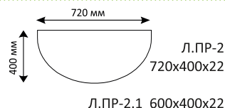
Л.ПР-2.1 600x400x22
