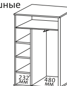
Л.ГБ-4 778x410x1975
