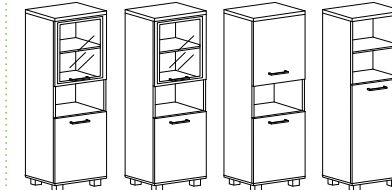
KSU-1.1 KSU-1.2 KSU-1.2R KSU-1.3 размеры 400x430x2060
