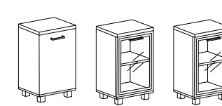
KSU-3.1 KSU-3.2 KSU-3.2R размеры 400x430x960
