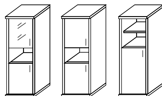
A.СУ-1.4 Л/Пр A.СУ-1.5 Л/Пр A.СУ-1.6 Л/Пр размеры 403x365x1975
