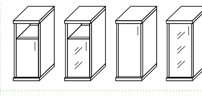
A.СУ-1.7 Л/Пр A.СУ-1.8 Л/Пр A.СУ-1.9 Л/Пр размеры 403x365x1975
