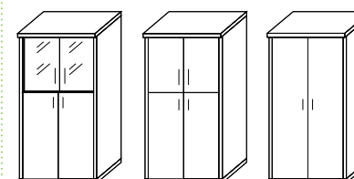
A.СУ-1.7 Л/Пр A.СУ-1.8 Л/Пр A.СУ-1.9 Л/Пр размеры 403x365x1975
