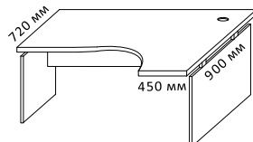
Л.СА-1 Л/Пр 1580x900x755 Л.СА-2 Л/Пр 1380x900x755
