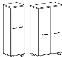
KG-1 600x430x2060 KG-2 800x430x2060
