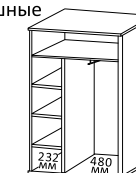
Л.ГБ-4 778x410x1975
