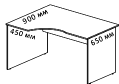
В.СА-2 Л 1400x900x755
