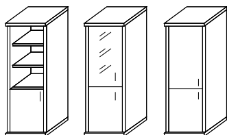
A.СУ-1.1 Л/Пр A.СУ-1.2 Л/Пр A.СУ-1.3 Л/Пр размеры 403x365x1975
