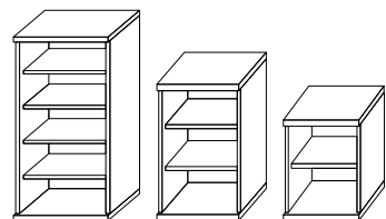
Л.СТ-1 778x410x1975 Л.СТ-2 778x410x1200 Л.СТ-3 778x410x823
